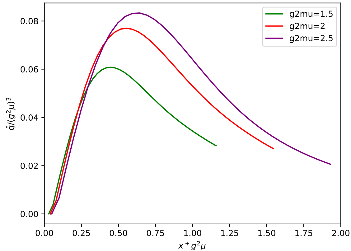
Jet quenching parameter
